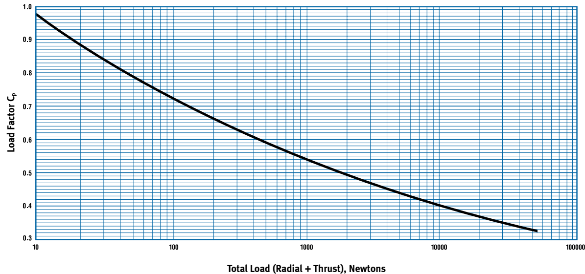
Fig. 19. Load factor Cp.
